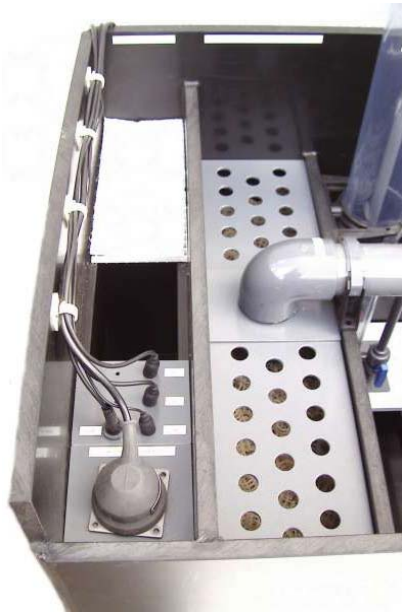
1.+2. Kammer mit Einlaufvlies, MSR- und Heizungshalter, Überlaufsieb für Rieselfilter, Zulauf vom Abschäumer
